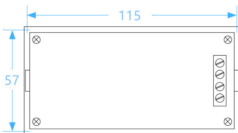
高度尺寸
