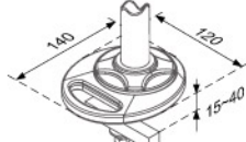
LA-526-1 Grommet Type
