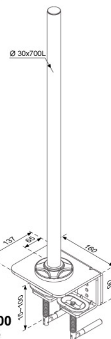
LA-502-700 Long Pole Grommet Type
