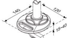
LA-527-1 Grommet Type
