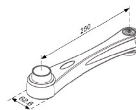
LA-513 Long Arm
