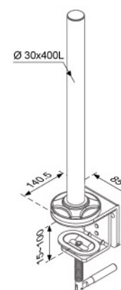
LA-502 Grommet Type
