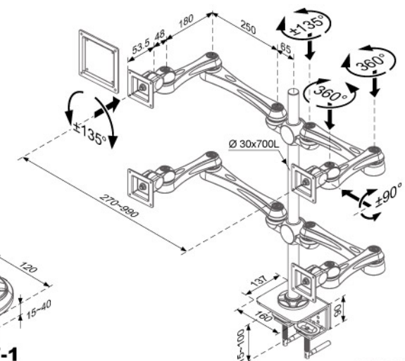
LA-517-1 unit:mm
