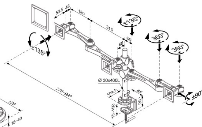
LA-516-1 unit:mm
