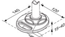
LA-525-1 Grommet Type
