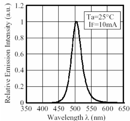
■ Spectrum
