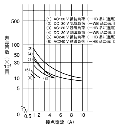
寿命曲線 (10 A 定格品のブレイク接点側)
