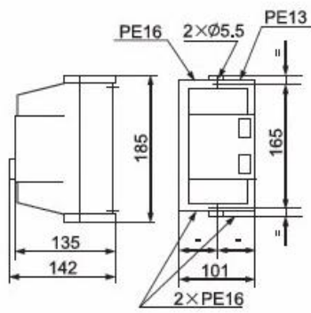
LE-D25~LE-D32
