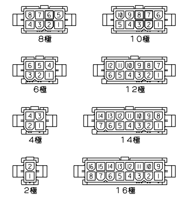
極数別レイアウト図 (SCALE : 1-1)
