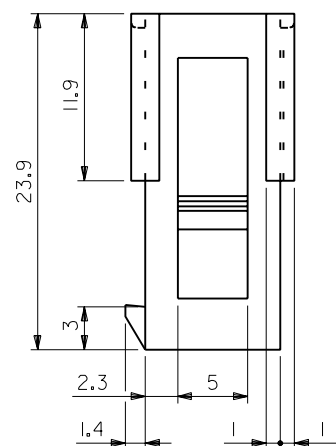
パネルスロット寸法 (パネル厚 0.8 - 2.0)
