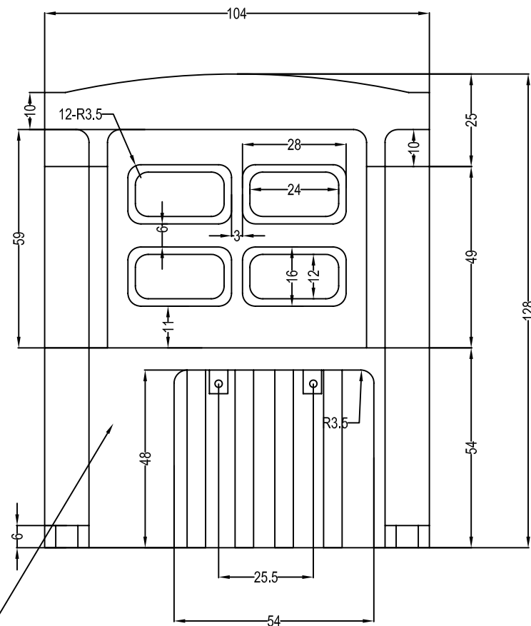
旋转90°侧面图
