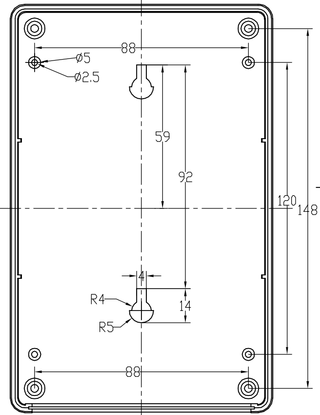
下盖正视图
