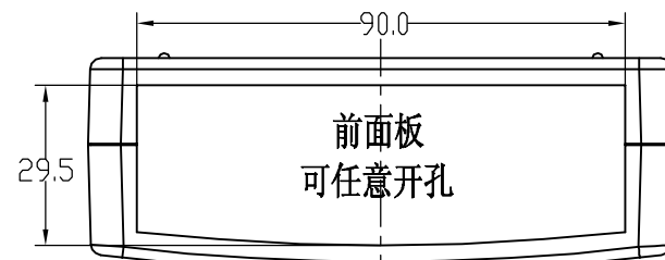
下盖正视图
