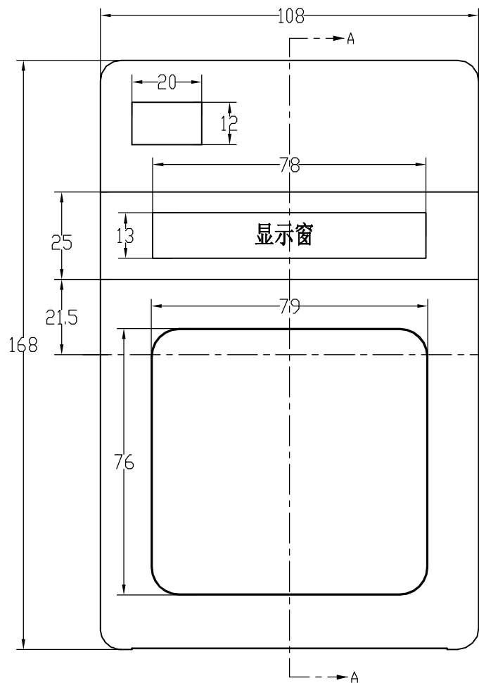
上盖正视图
