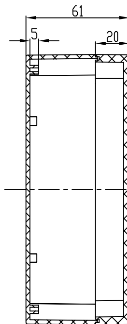
C-C
