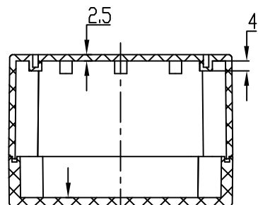
D-D
